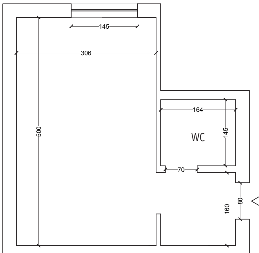
PIANTA DELLA STANZA TIPO SCALA 1:50
